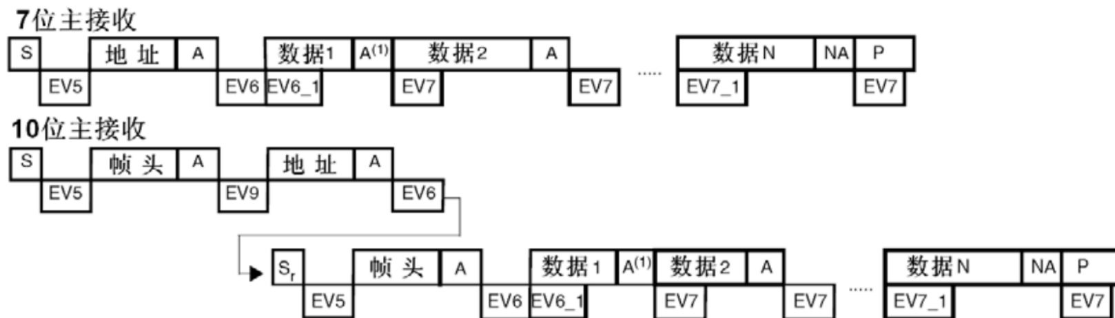
图246 主接收器传送序列图
