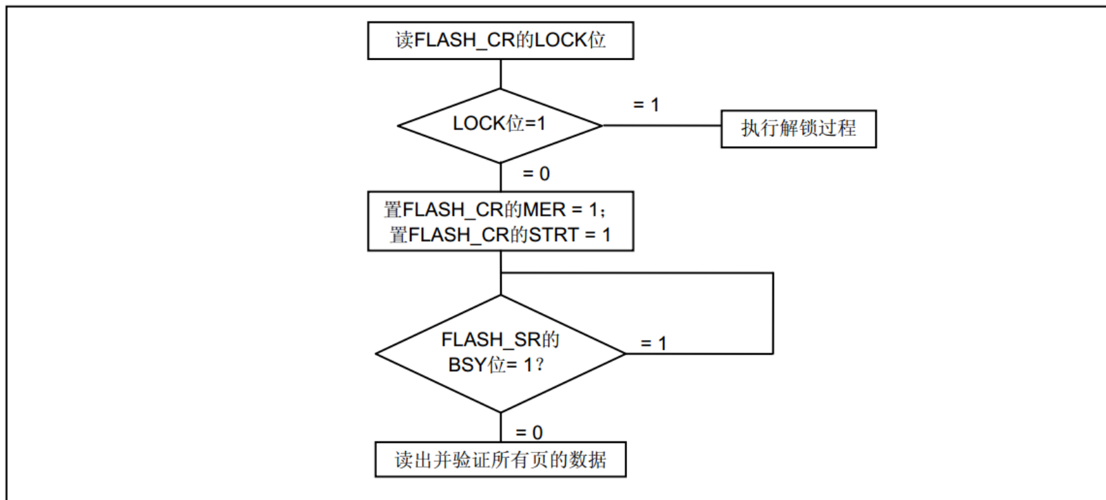
图三 闪存全擦除过程
