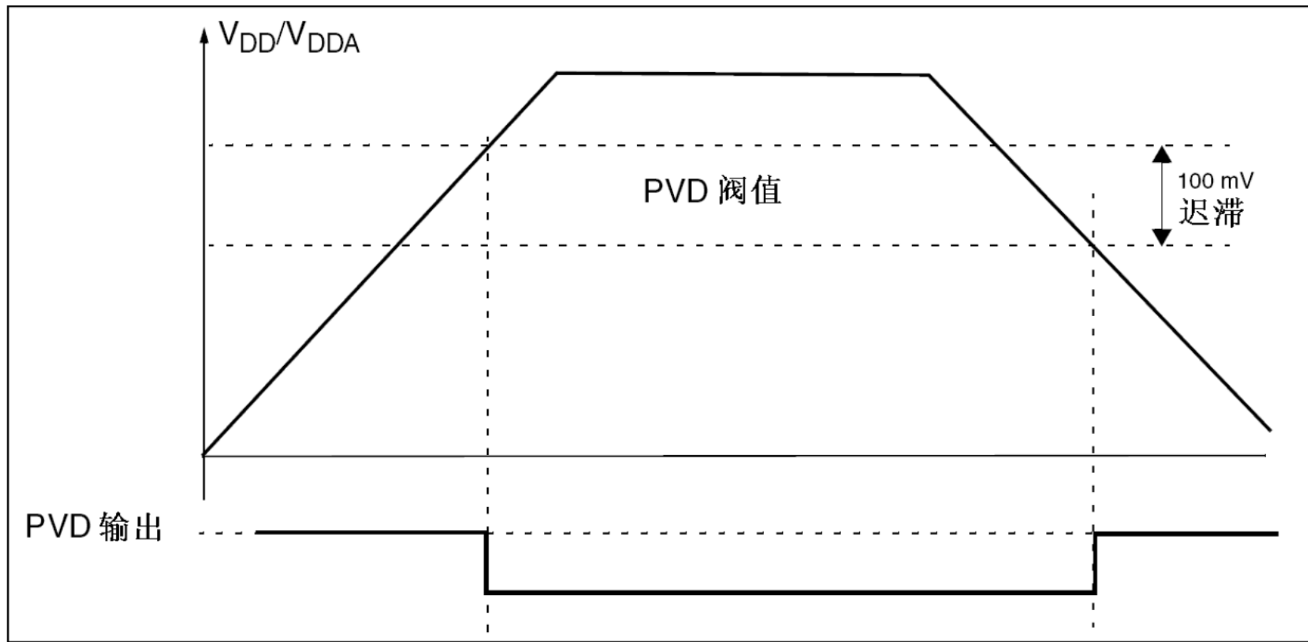
图6 PVD的门限
