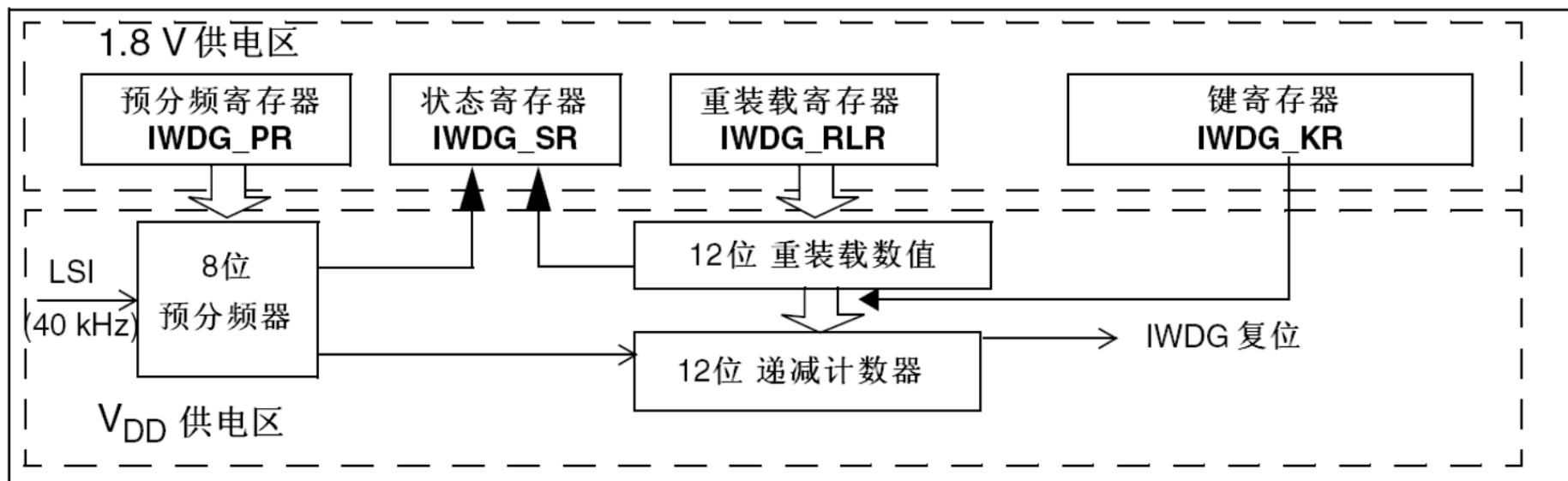
图157 独立看门狗框图
