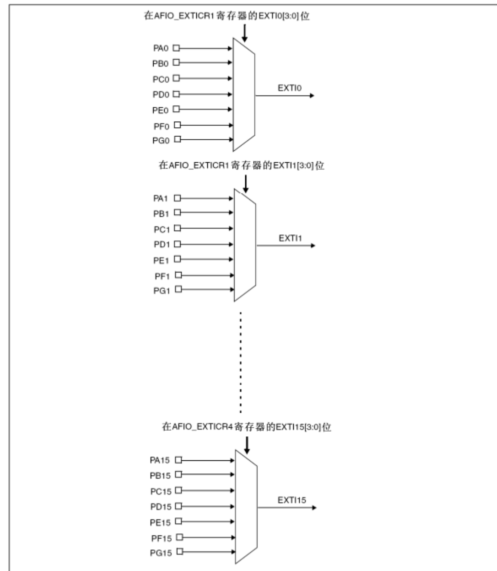
图20 外部中断通用I/O映像
