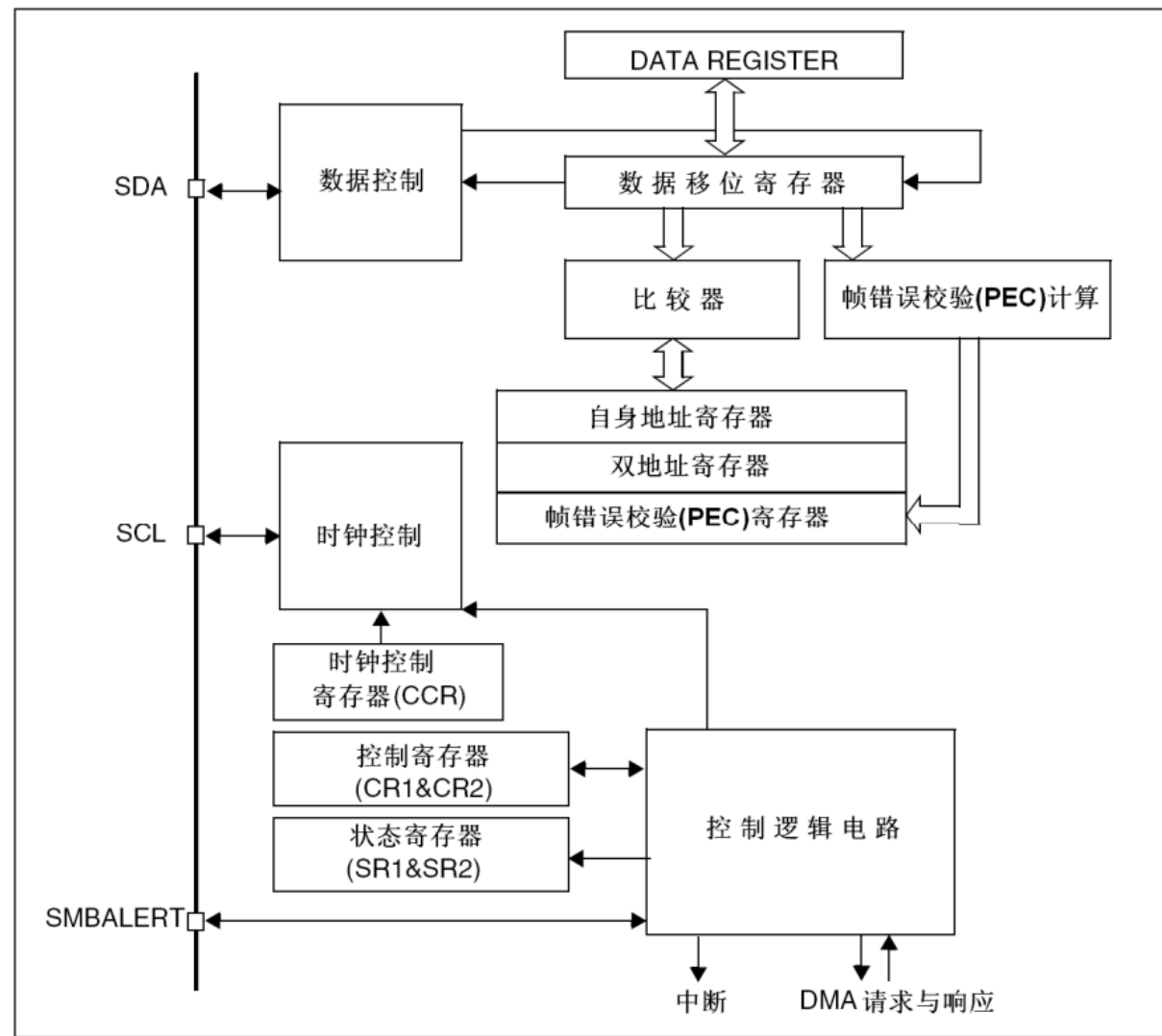
图242 I 2 C的功能框图
