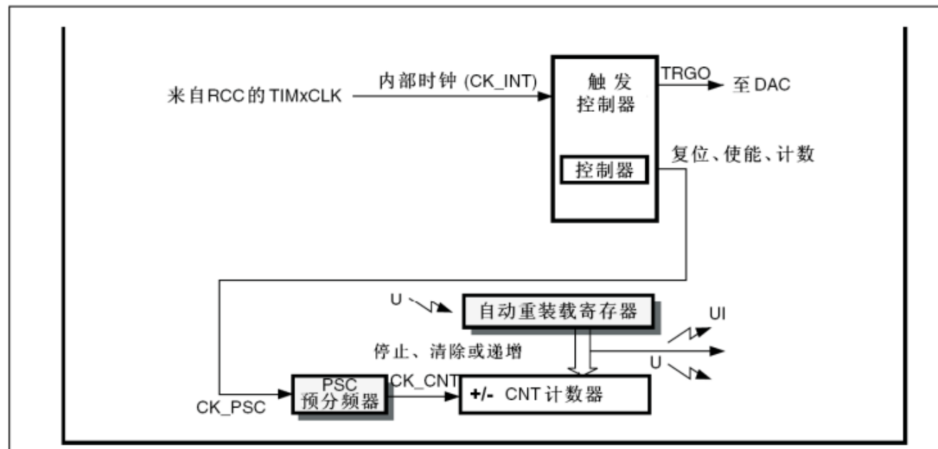
图144 基本定时器框图
