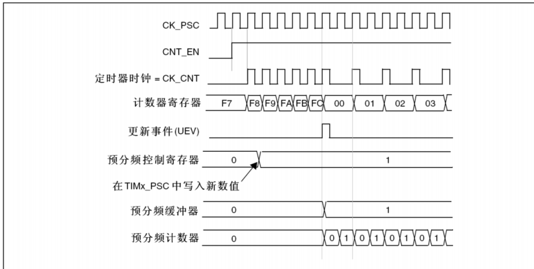
图99 当预分频器的参数从1变到2时，计数器的时序图
