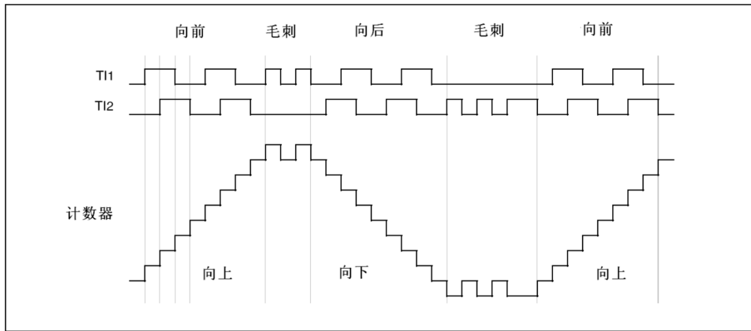
图132 编码器模式下的计数器操作实例
