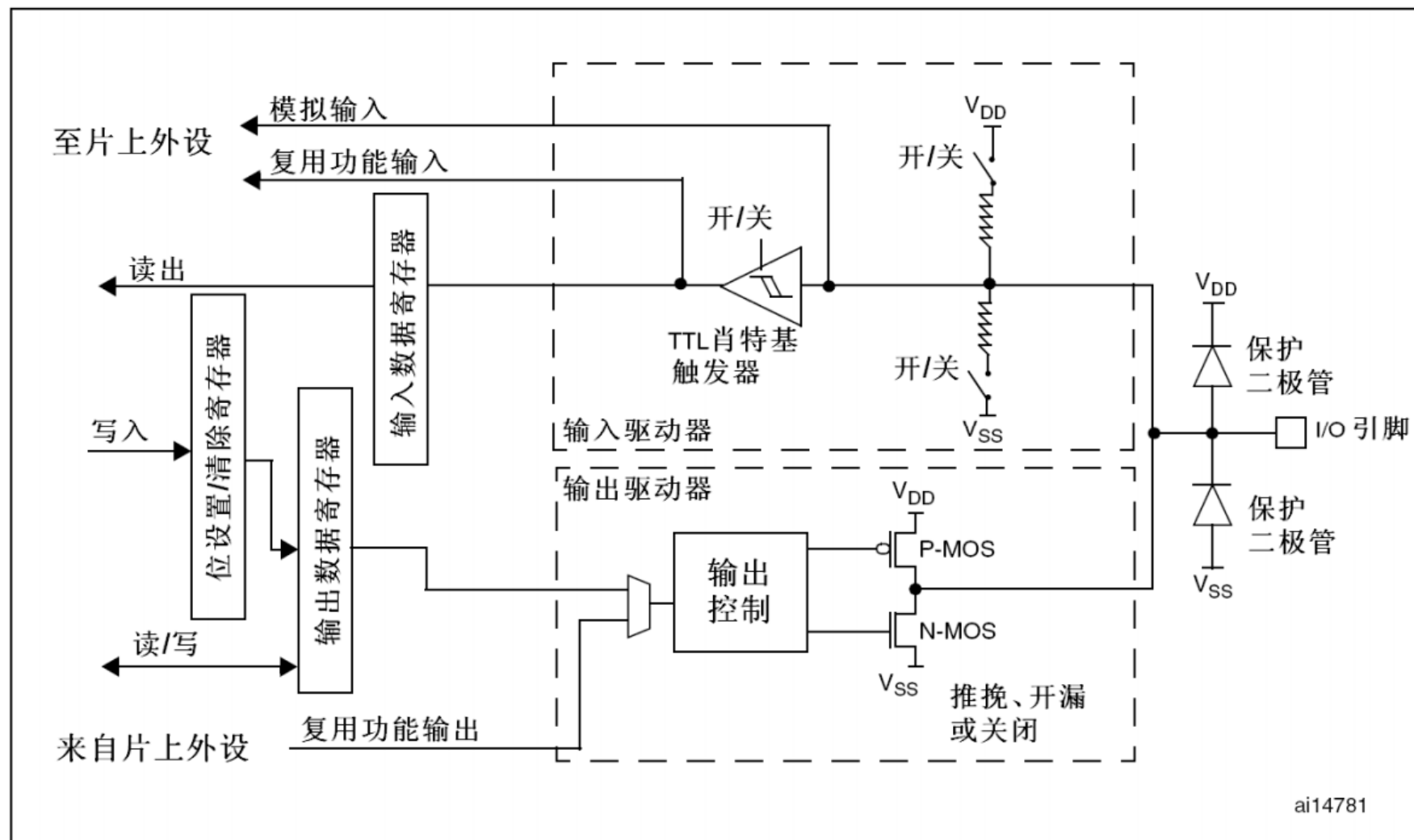
图13 I/O端口位的基本结构
