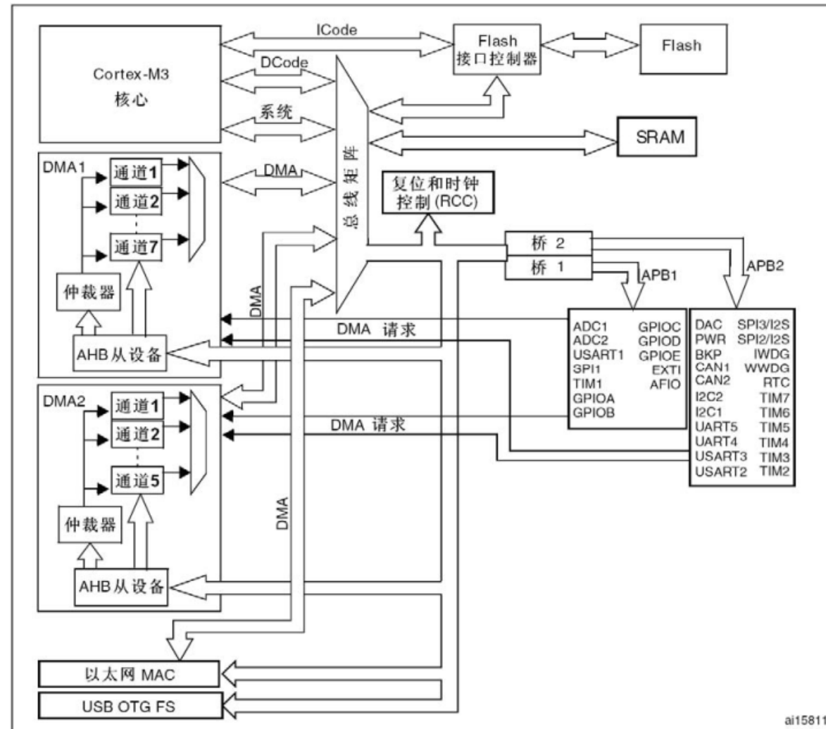
图21 DMA框图
