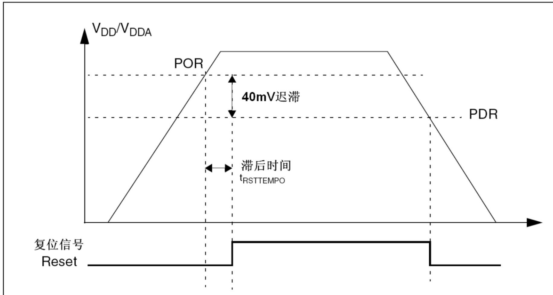
图5 上电复位和掉电复位的波形图
