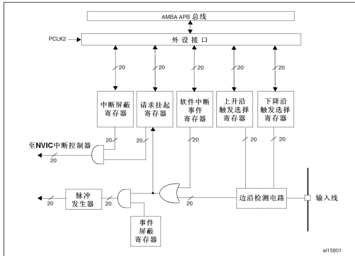
图19 外部中断/事件控制器框图
