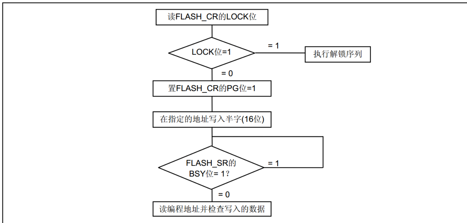
图一 编程过程
