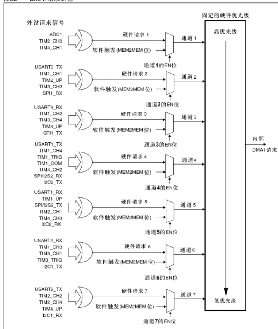
图22 DMA1请求映像
