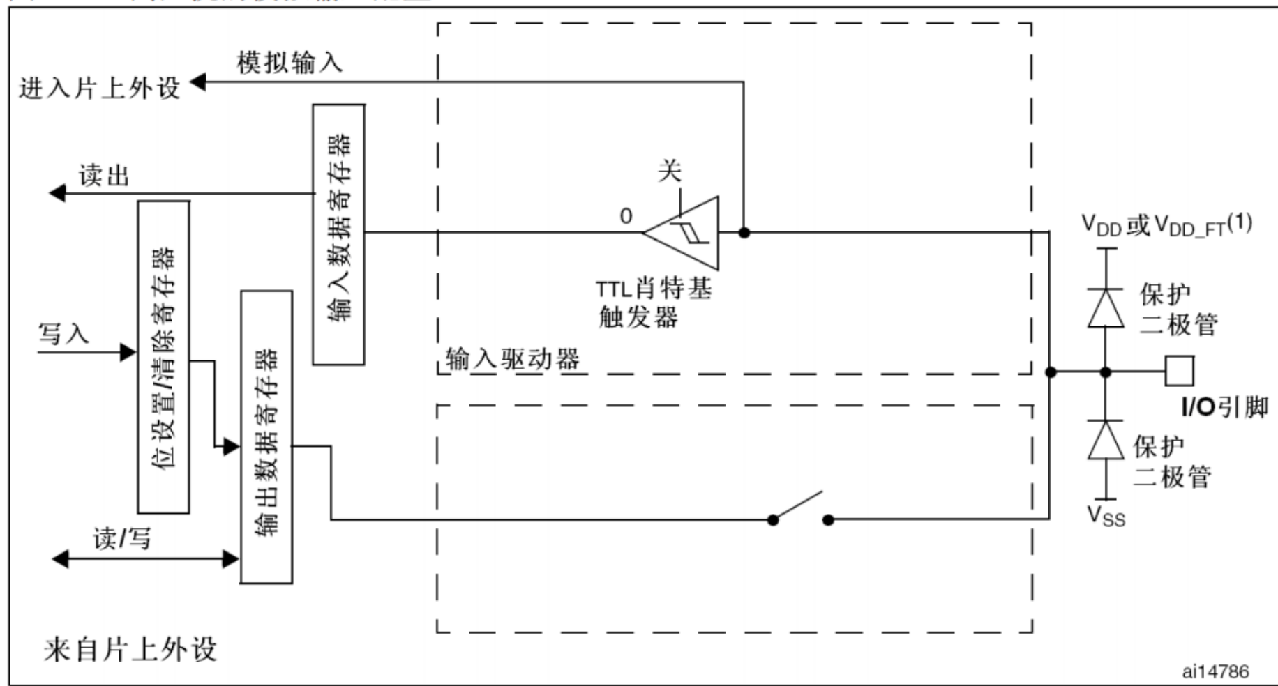
图18 高阻抗的模拟输入配置
