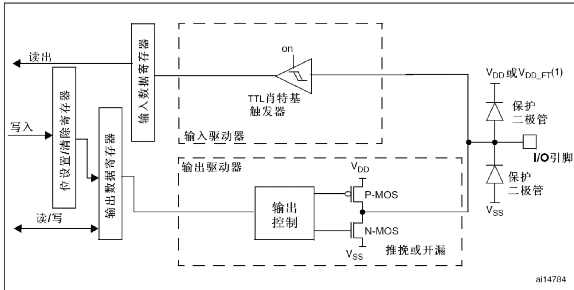
图16 输出配置
