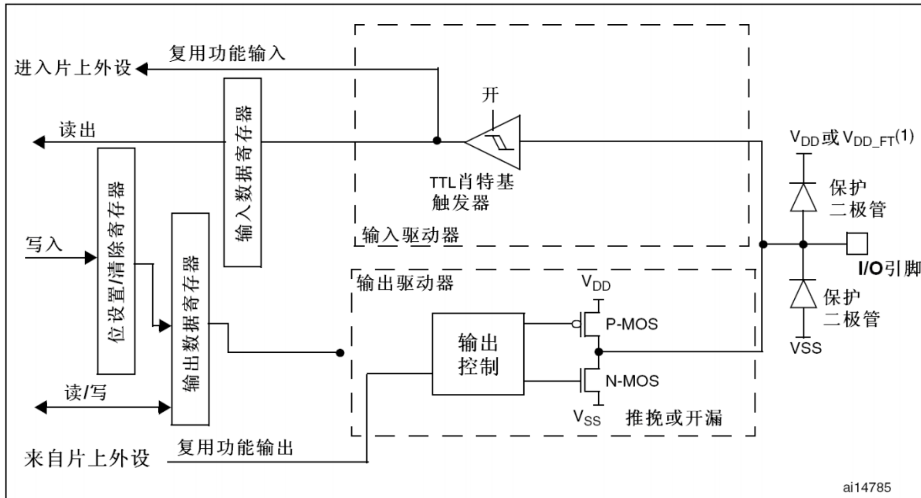
图17 复用功能配置
