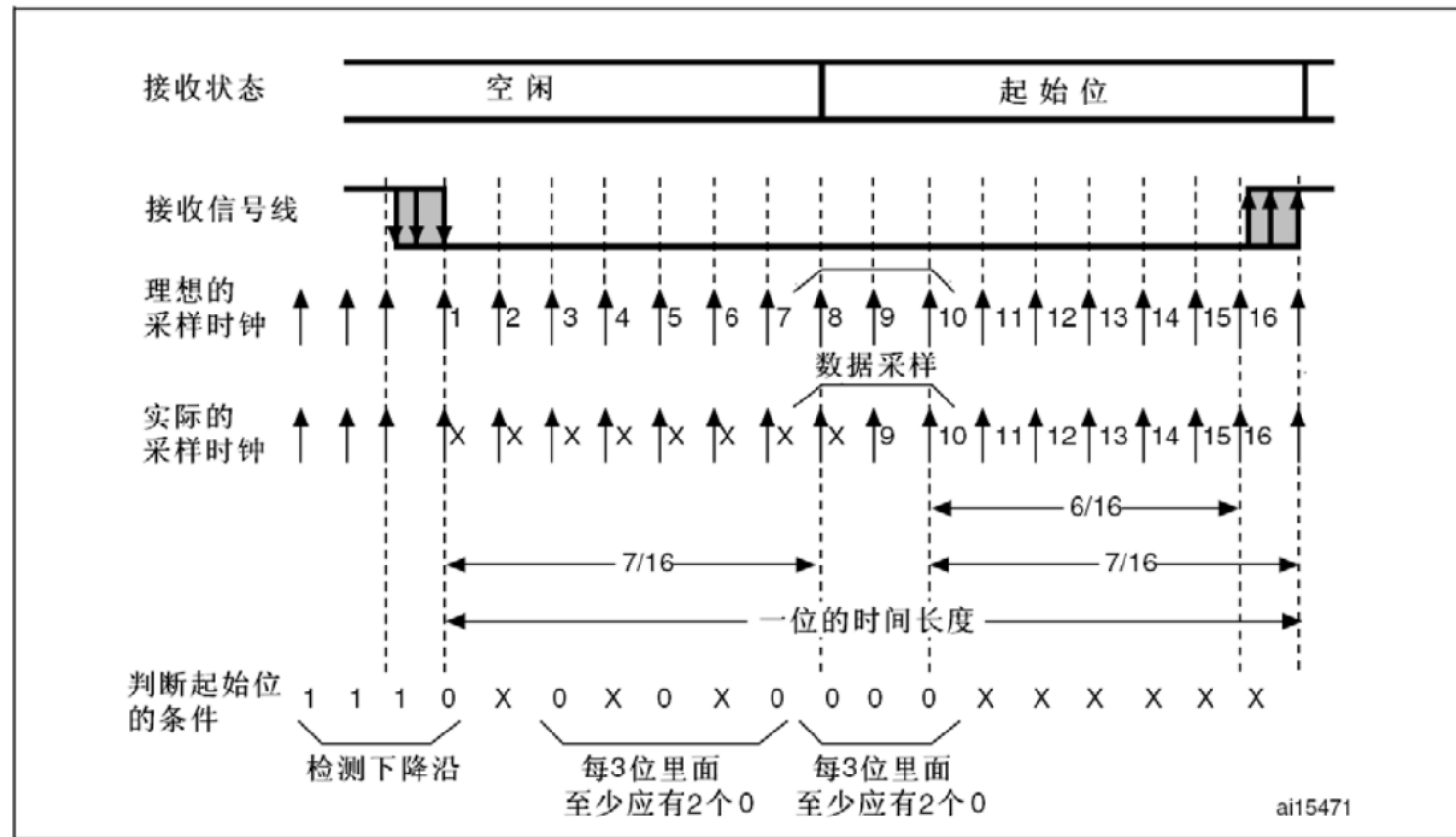
图252 起始位侦测
