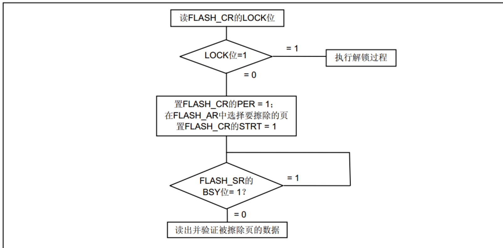
图二 闪存页擦除过程
