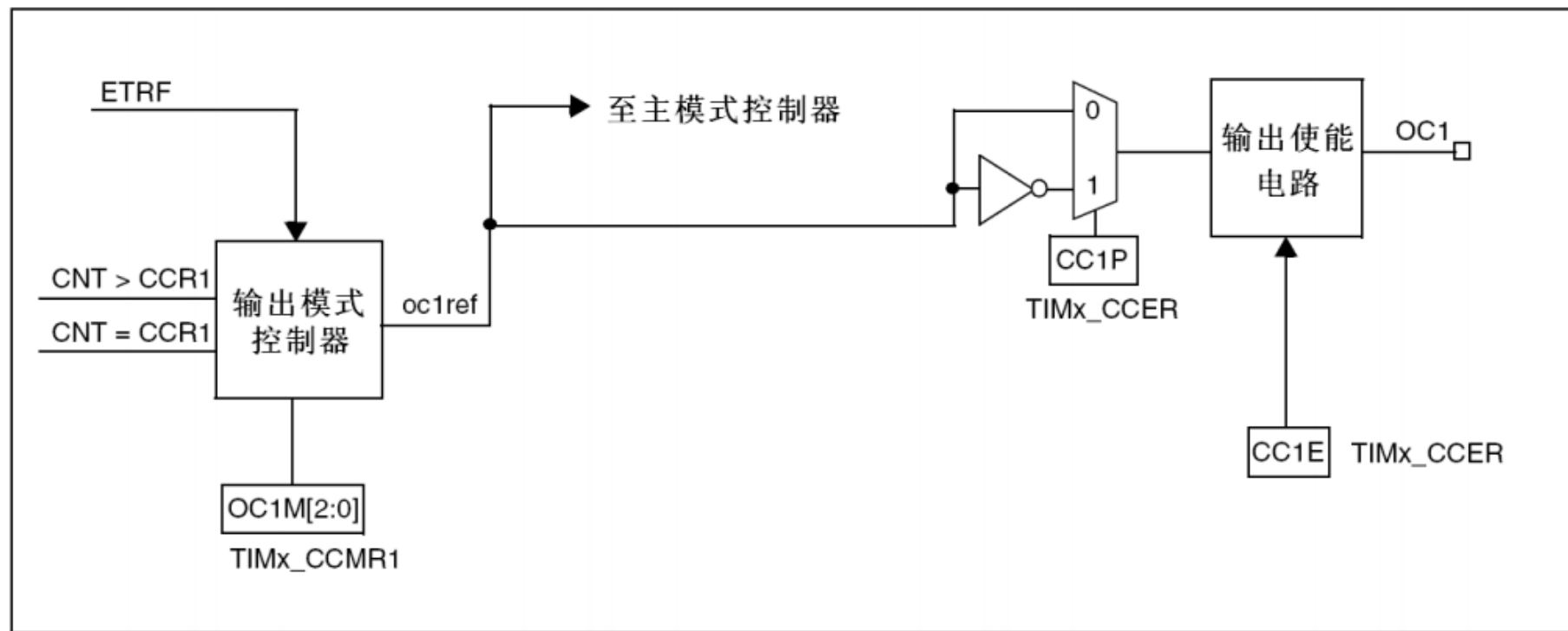
图125 捕获/比较通道的输出部分(通道1)
