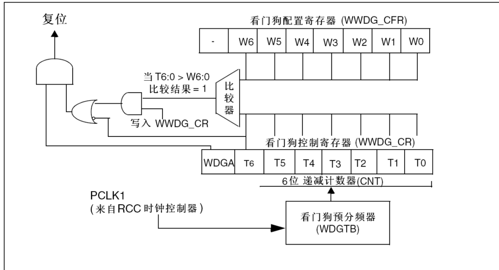
图158 看门狗框图
