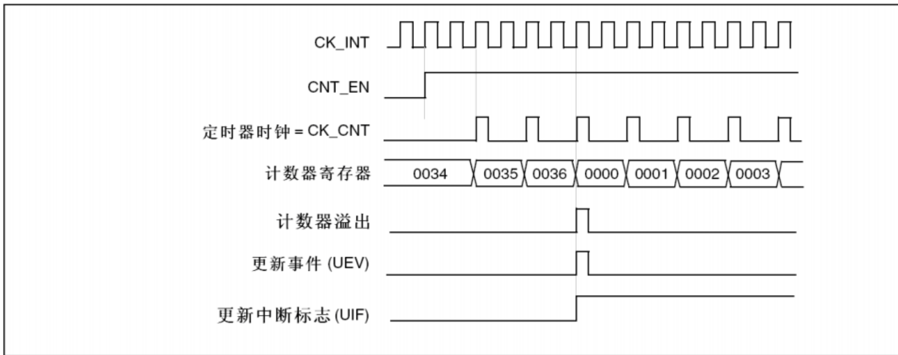
图102 计数器时序图，内部时钟分频因子为2
