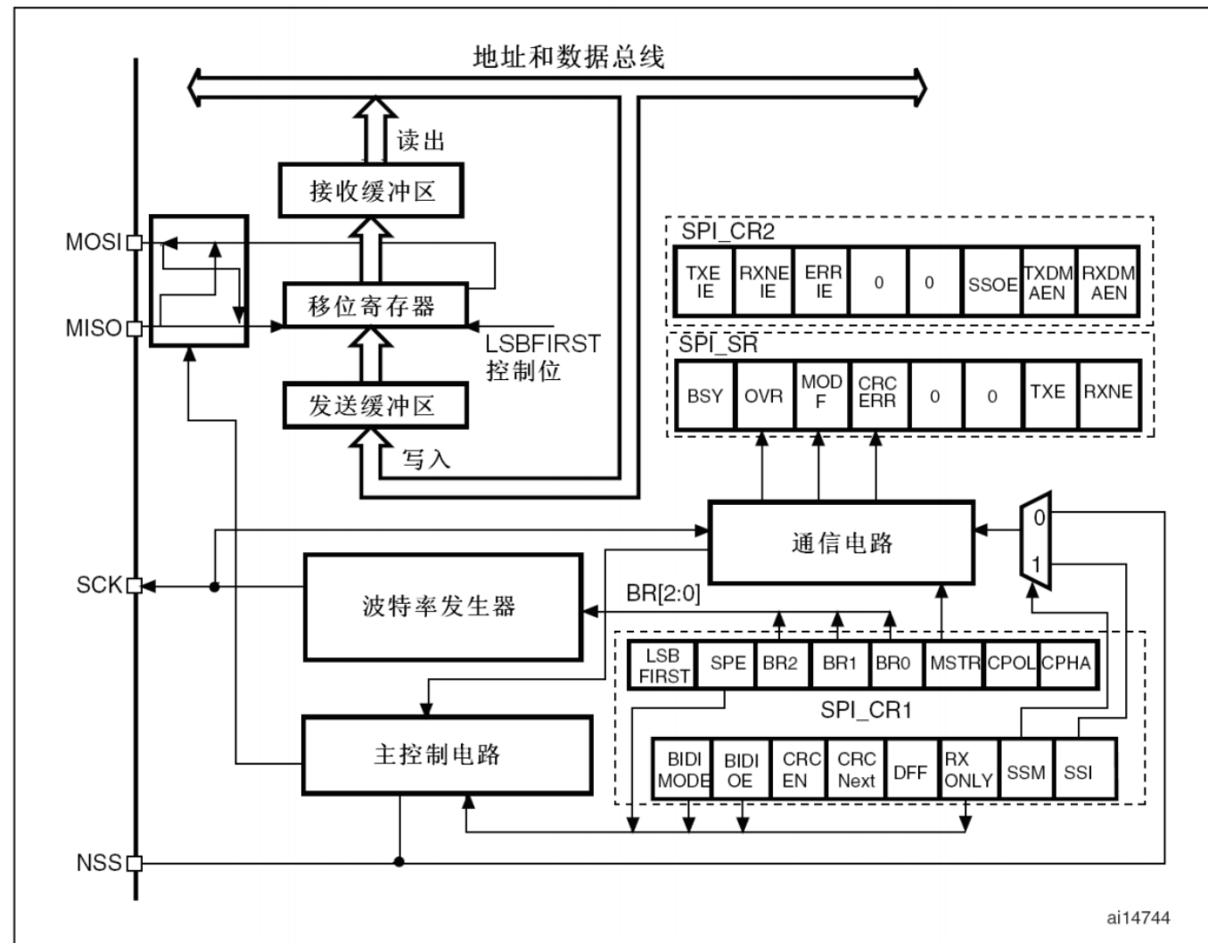
图209 SPI框图
