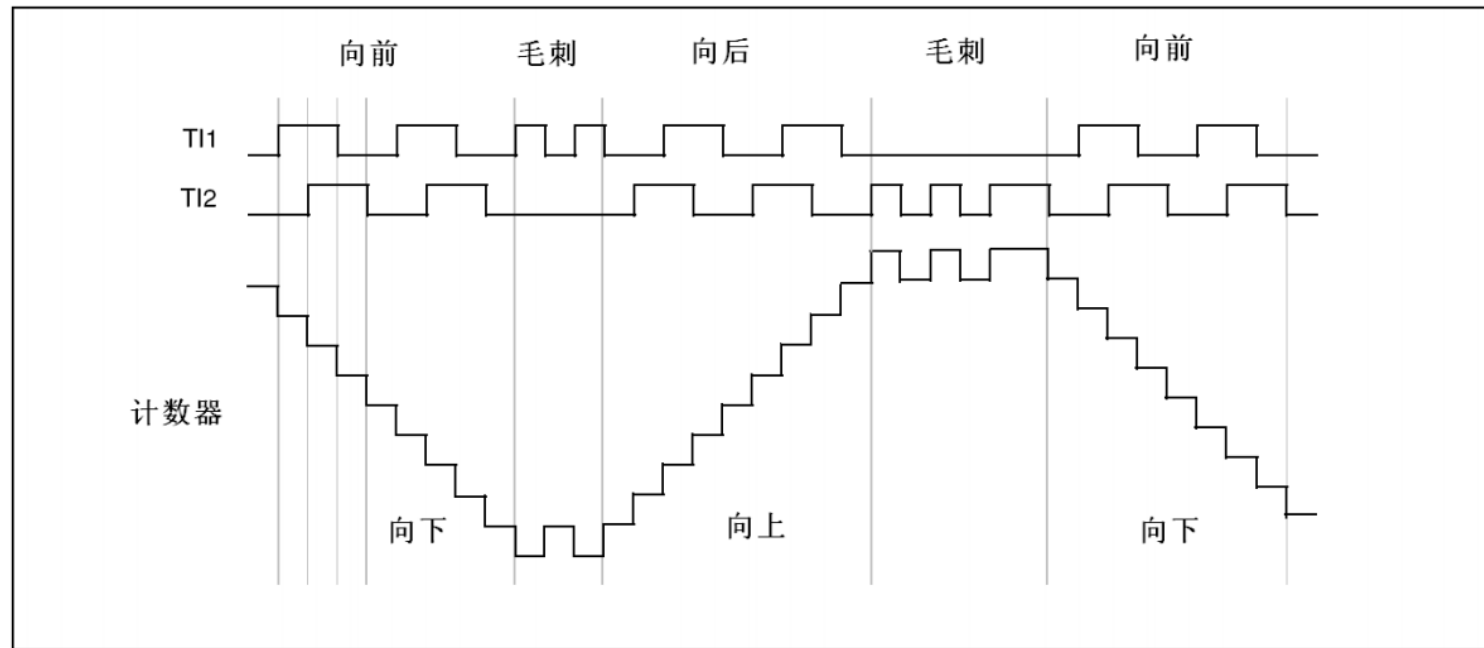
图133 IC1FP1反相的编码器接口模式实例
