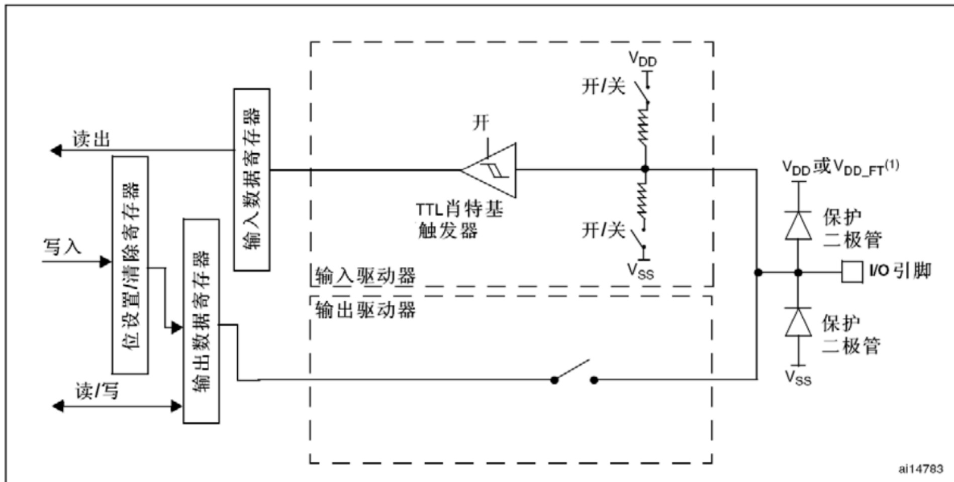
图15 输入浮空/上拉/下拉配置
