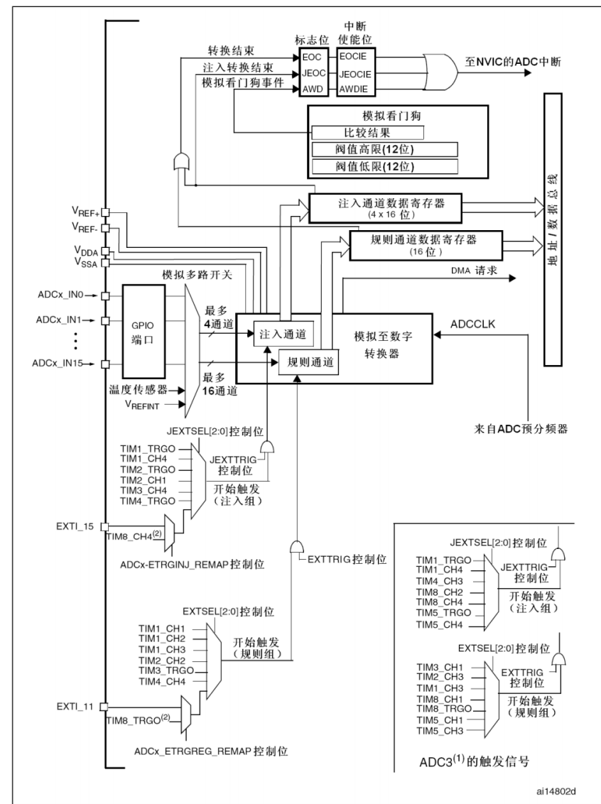
图24 单个ADC框图
