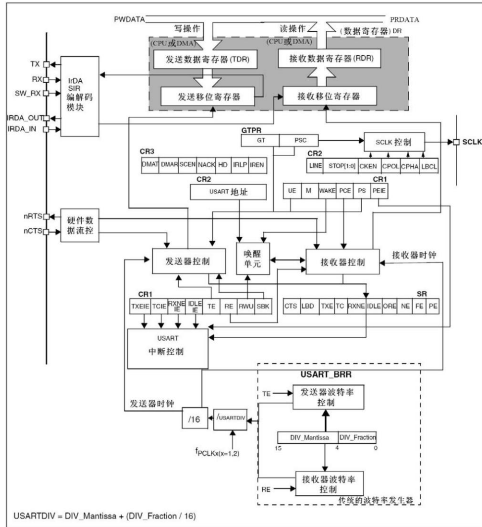
图248 USART框图
