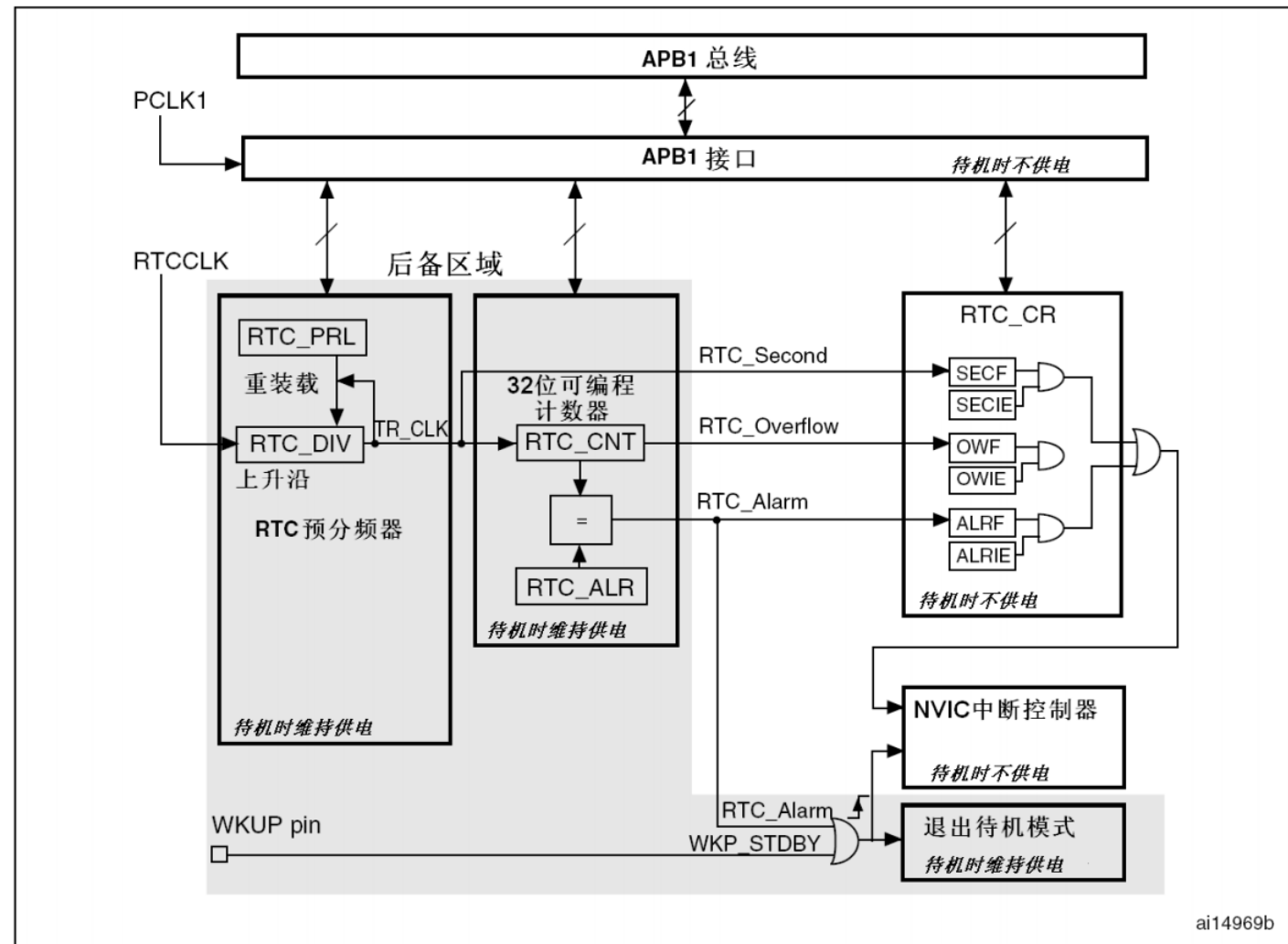
图154 简化的RTC框图
