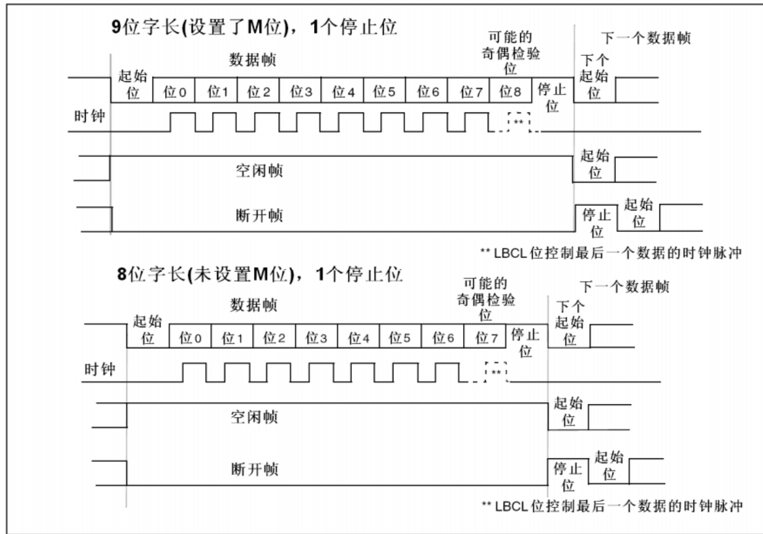
图249 字长设置
