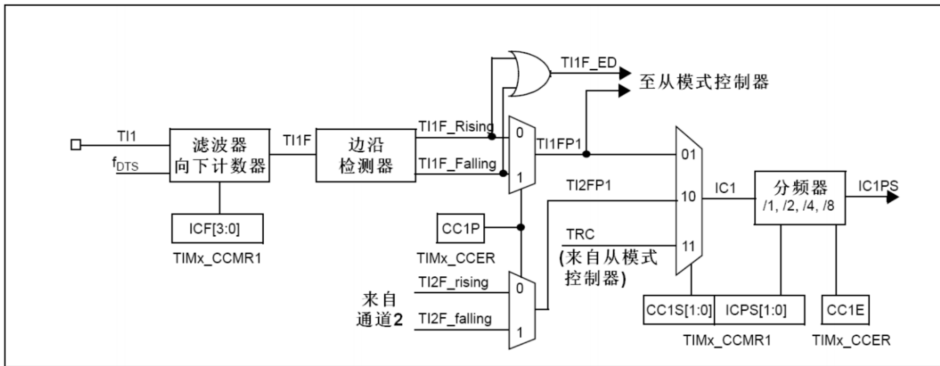
图123 捕获/比较通道(如：通道1输入部分)
