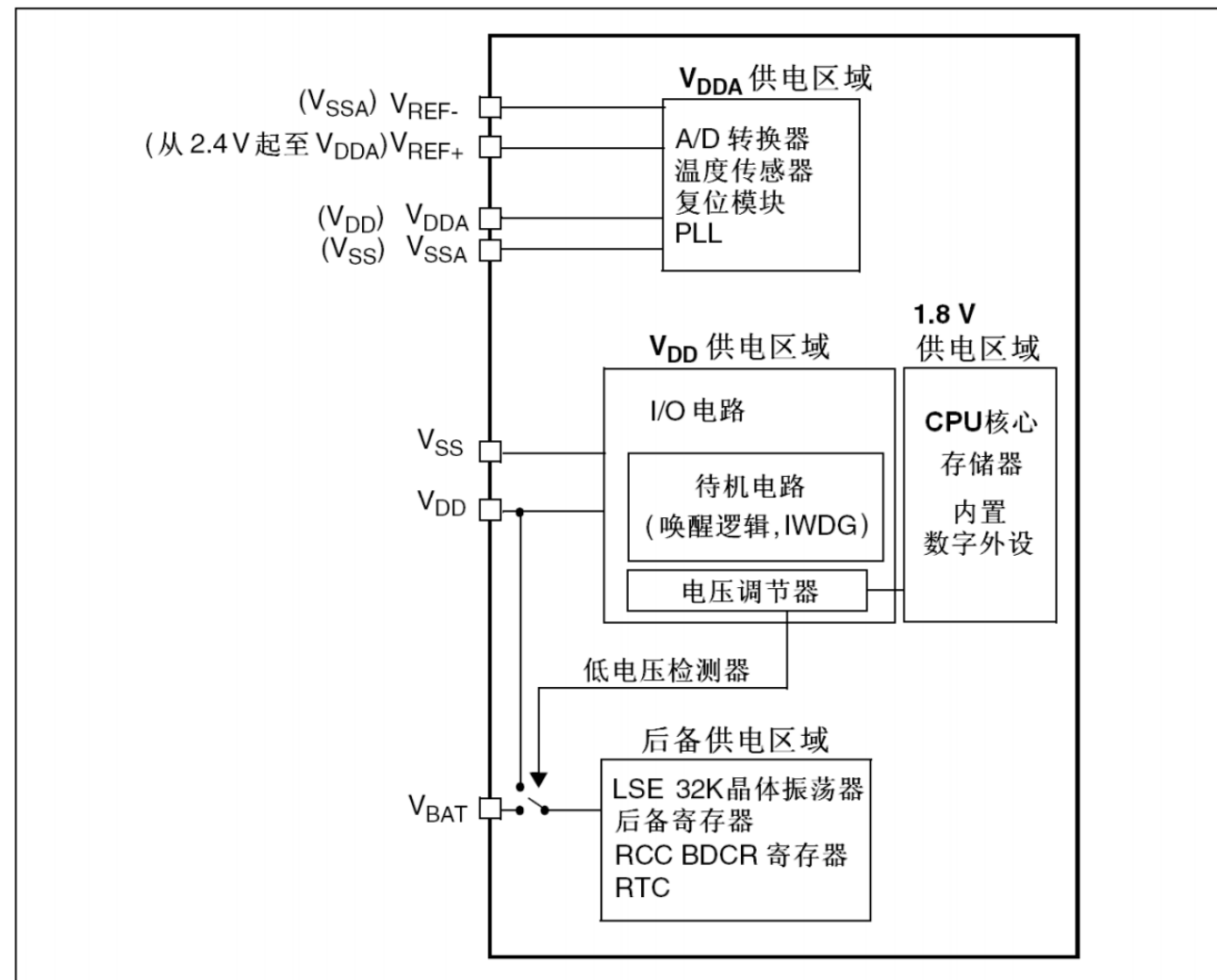
图4 电源框图
