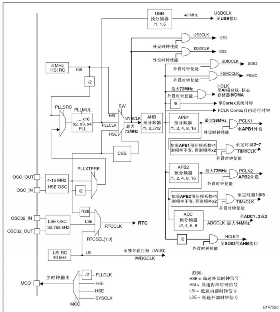
图8 时钟树
