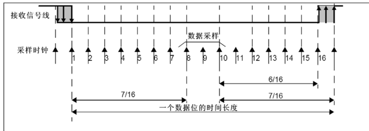
图253 检测噪声的数据采样
