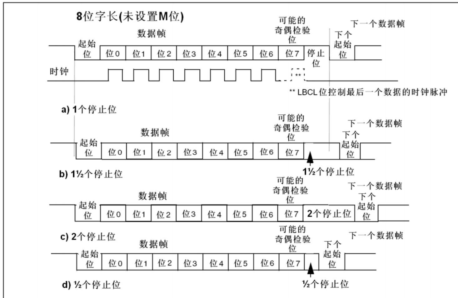
图250 配置停止位
