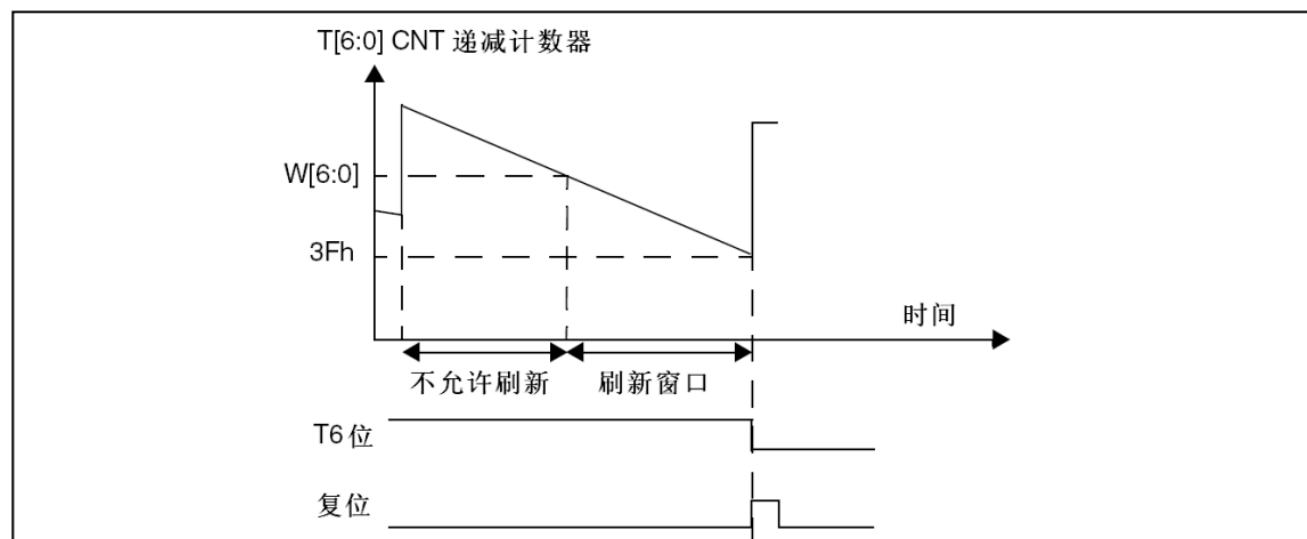
图159 窗口看门狗时序图
