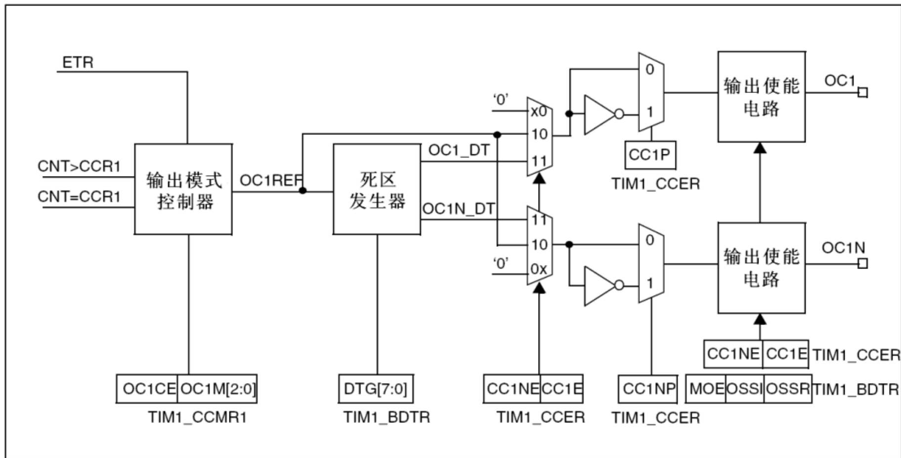
图78 捕获/比较通道的输出部分(通道1至3)
